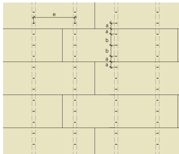
Abbildung 8: Klammerabstände im Feldbereich
