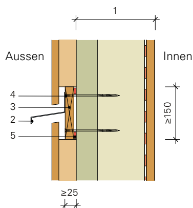
a) Füllholz vor Aussendämmung mit Brandschutzfugenbänder
