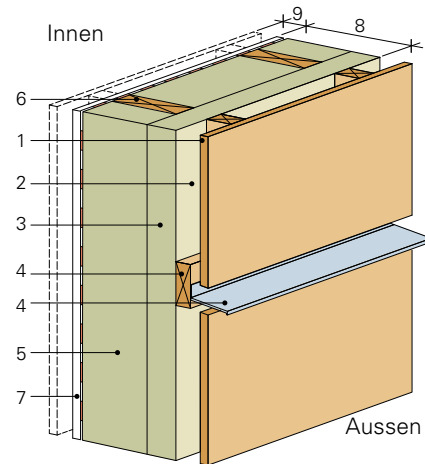
Abbildung 10: Nichttragende Aussenwandkonstruktion mit 30 Minuten Feuerwiderstand
