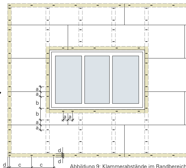
Abbildung 9: Klammerabstände im Randbereich
